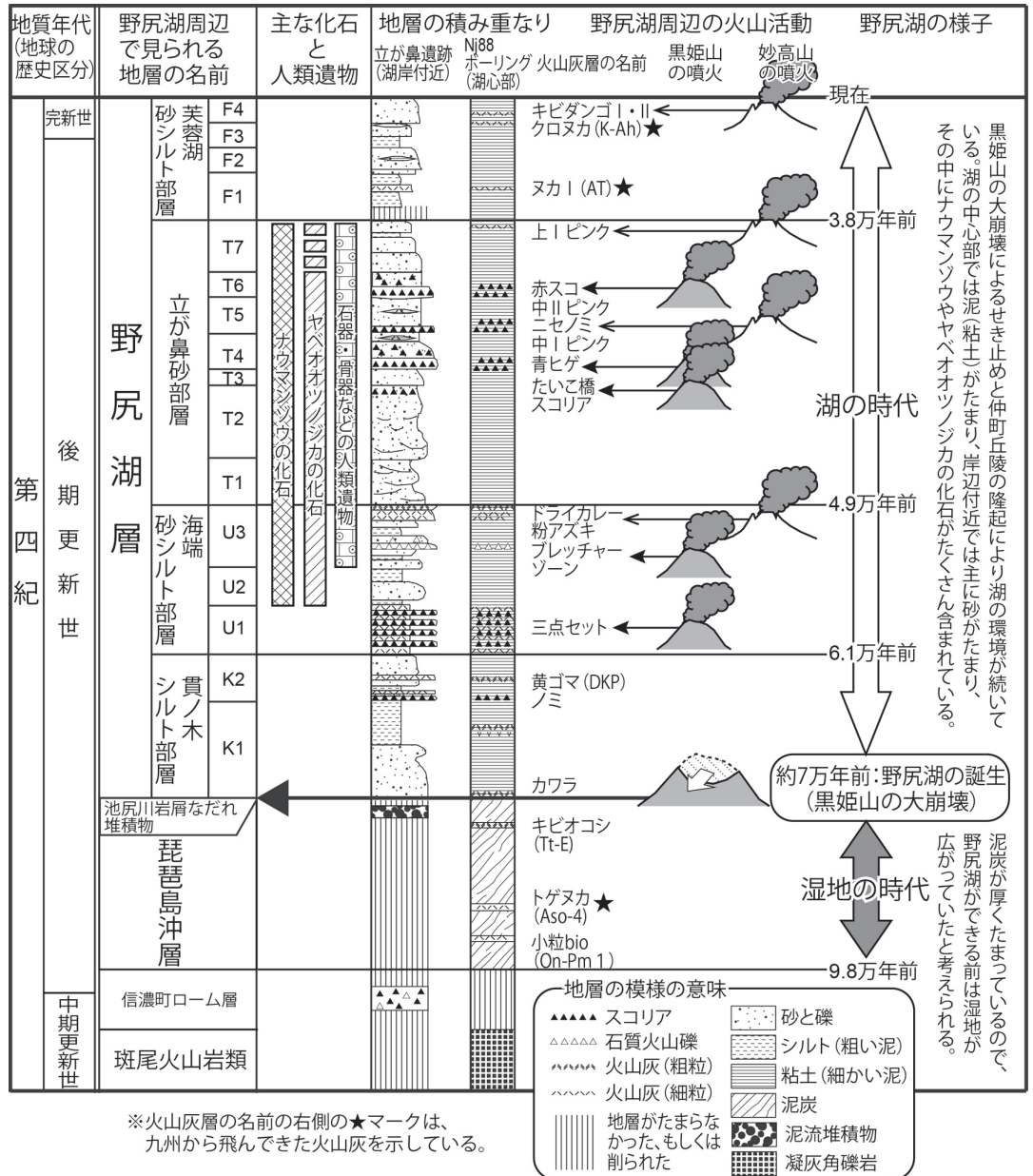
野尻湖層の層序（野尻湖のナウマンゾウより）
